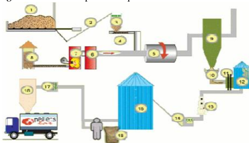
Figura 5: Etapas esquematizadas de Produção dos pellets
